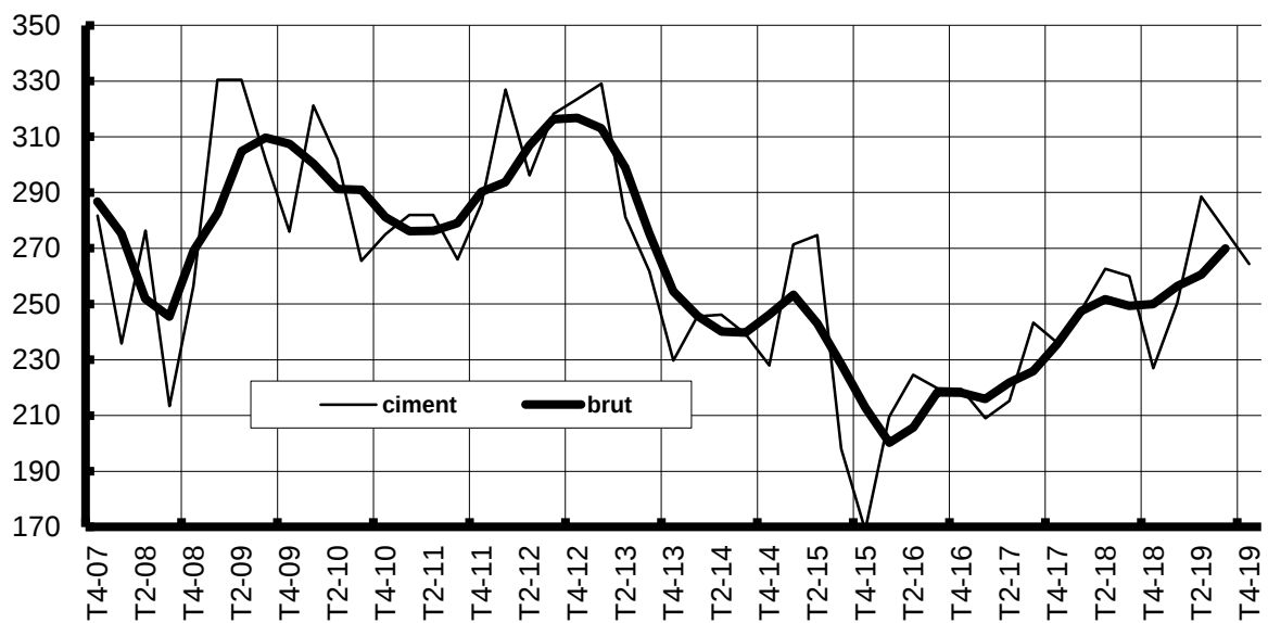
CIMENT (en milliers de tonnes)
