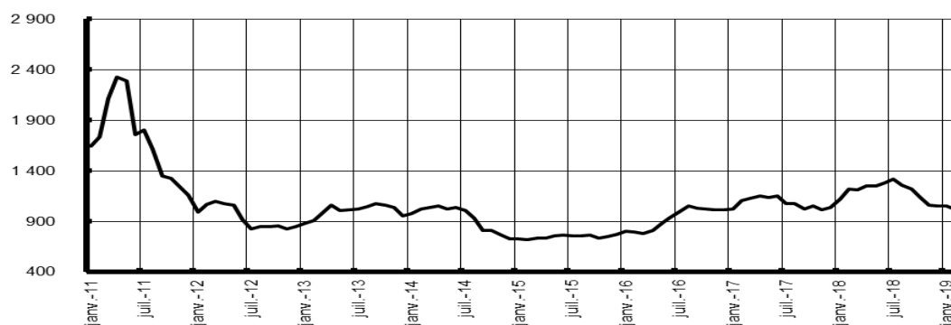
Cours du coton (FCFA / Kg)
