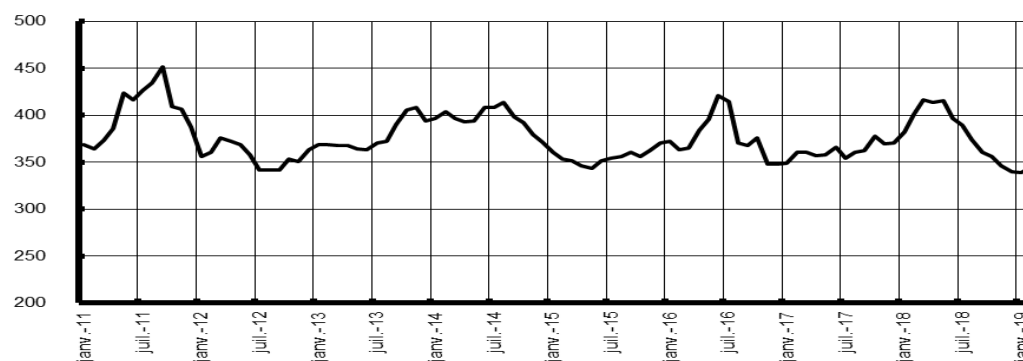
Cours du bois scié (1 000 FCFA / M 3 )
