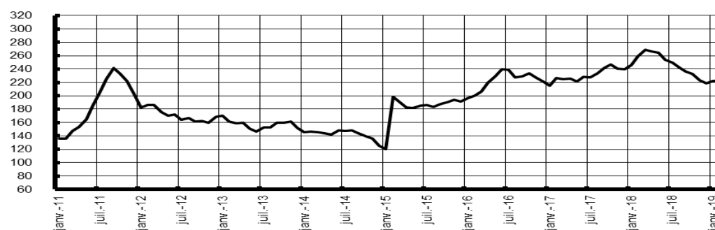
Cours du bois de grume (1 000 FCFA / M 3 )
