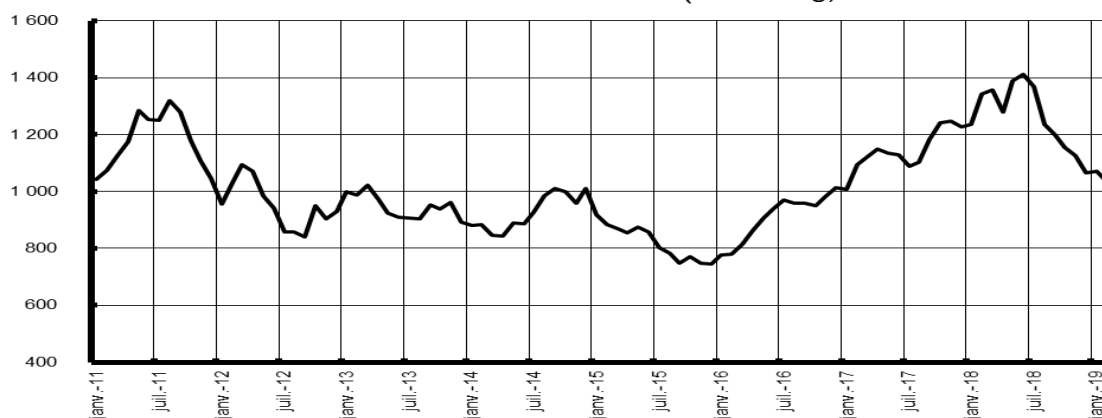
Cours de l'aluminium (FCFA / Kg)
