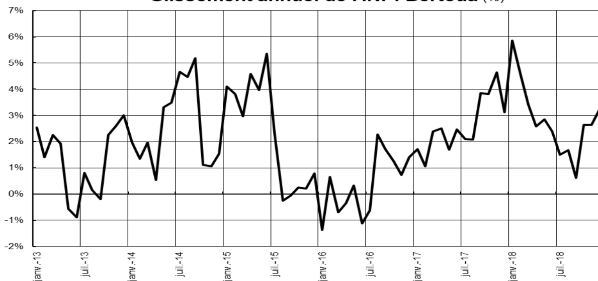
Glissement annuel de l'INP: Bertoua (%)
