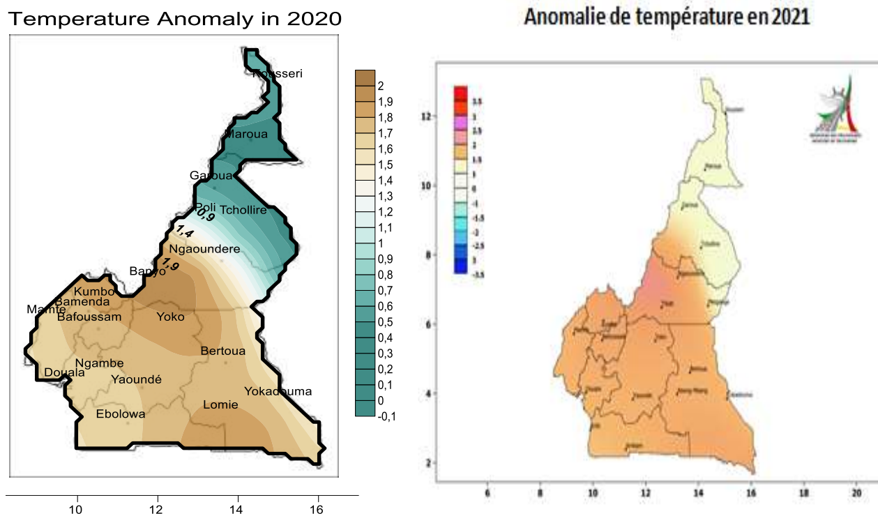
Figure 3- 6 : Anomalie de température en 2020 et 2021
