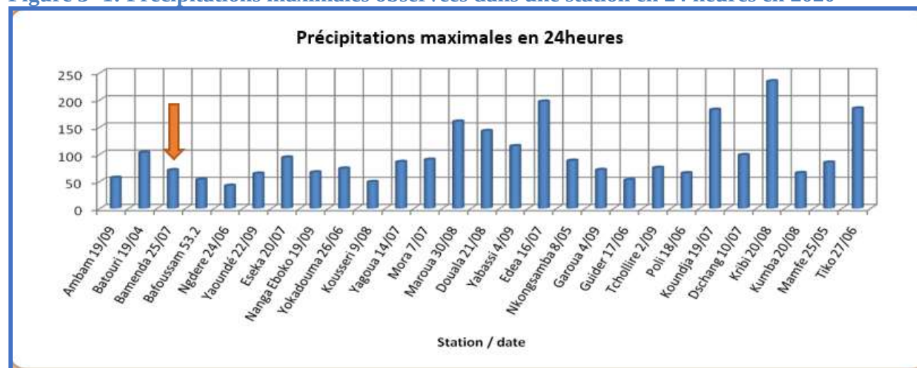
Figure 3- 1: Précipitations maximales observées dans une station en 24 heures en 2020
