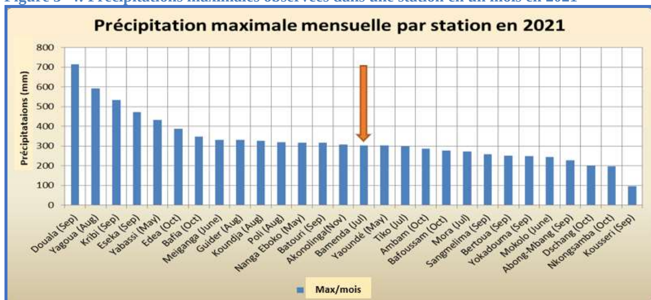
Figure 3- 4: Précipitations maximales observées dans une station en un mois en 2021
