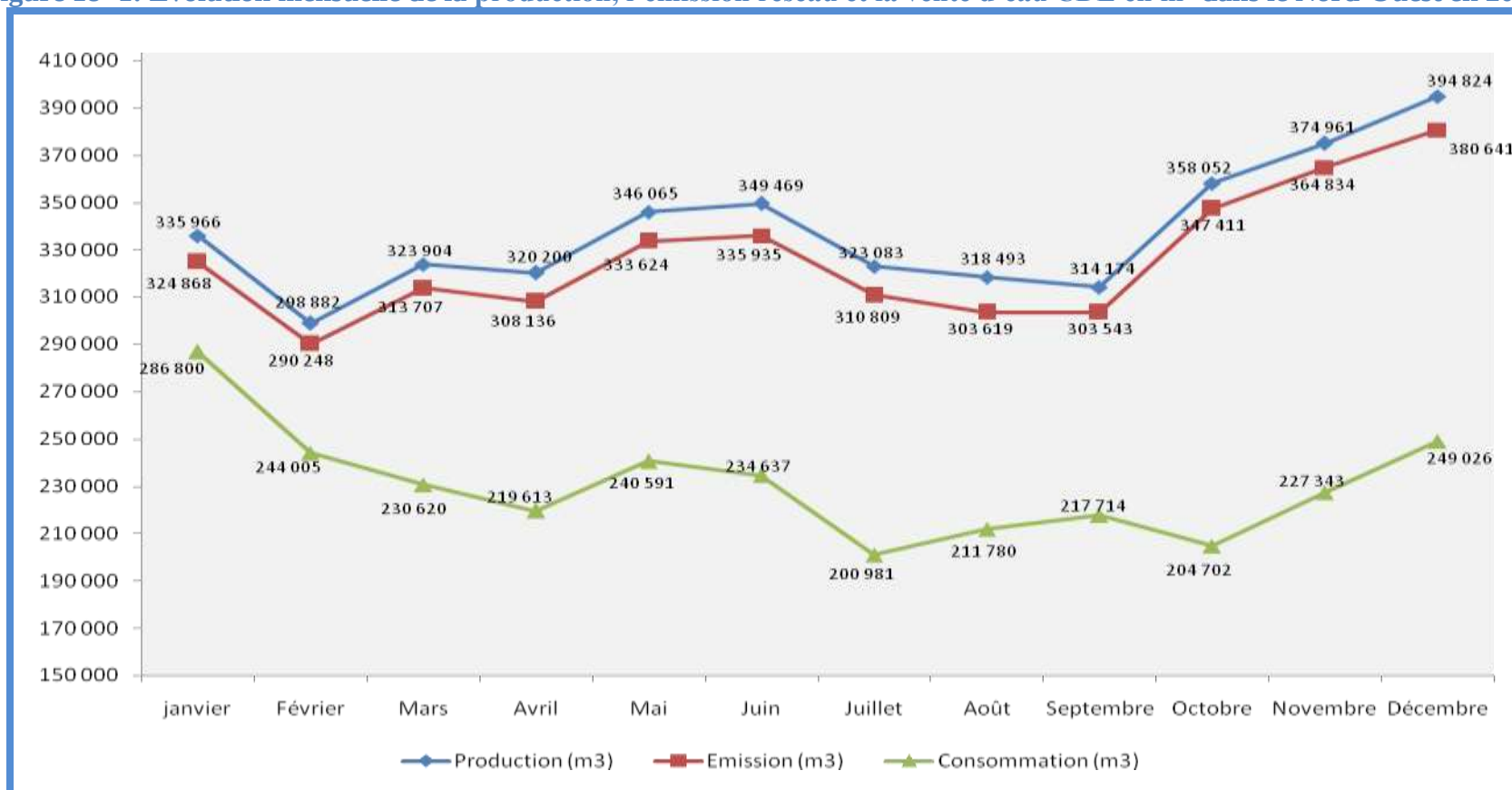
Figure 18- 1: Evolution mensuelle de la production, l'émission réseau et la vente d'eau CDE en m 3 dans le Nord-Ouest en 2016
