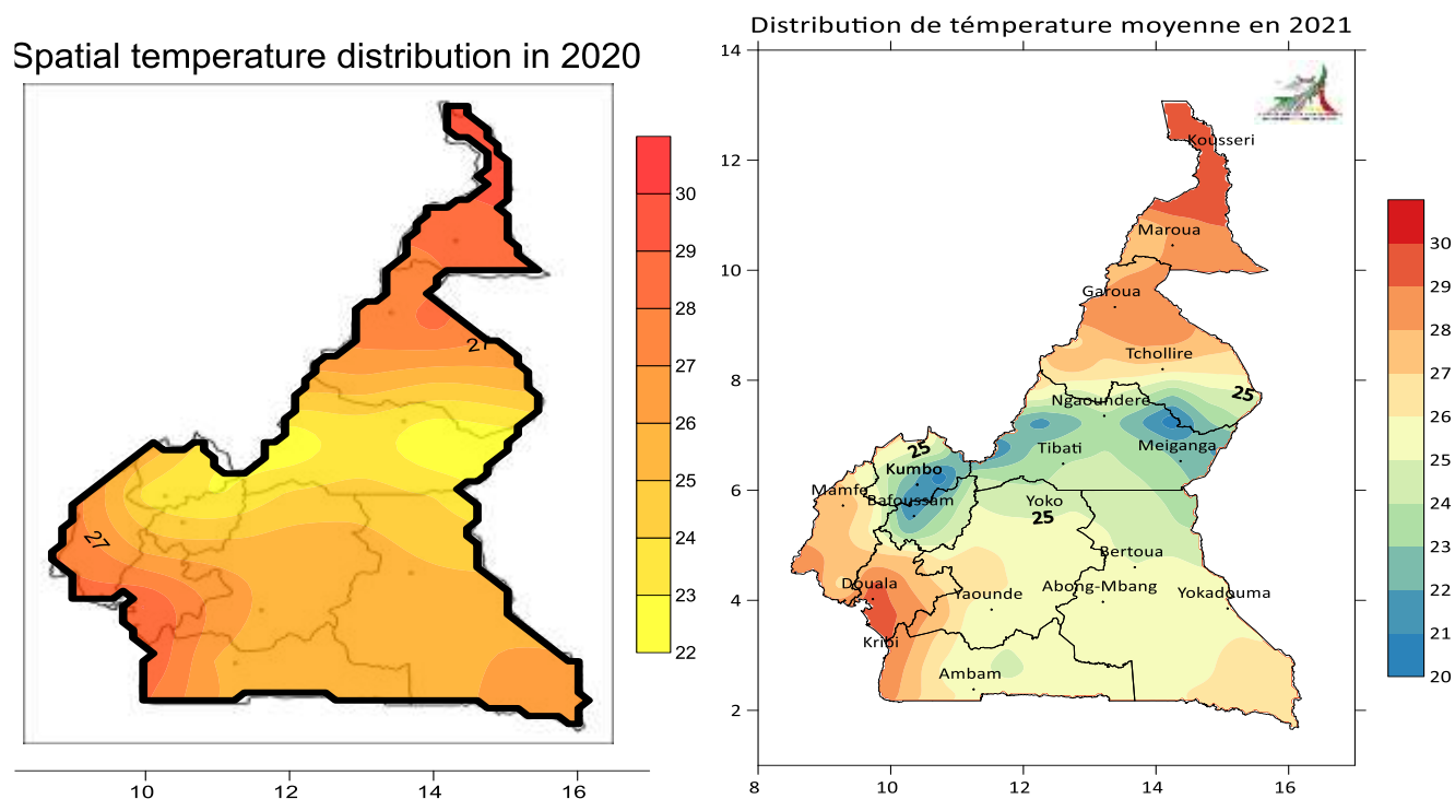
Figure 3- 5 : Température moyenne en 2020 et 2021
