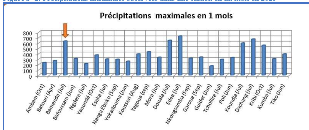
Figure 3- 2: Précipitations maximales observées dans une station en un mois en 2020
