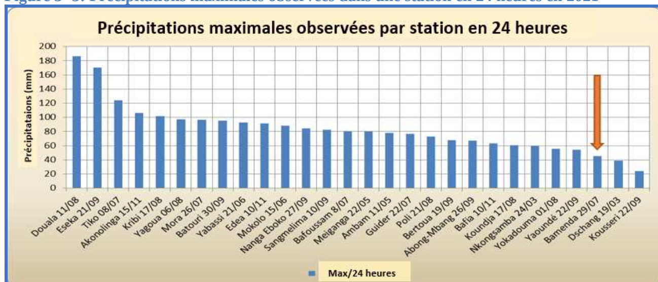
Figure 3- 3: Précipitations maximales observées dans une station en 24 heures en 2021
